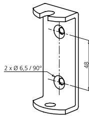
Markisenlager
