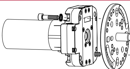
Markisenlager
