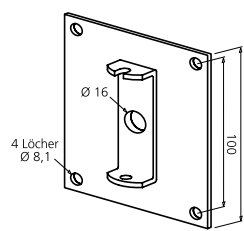
Rolltorlager
