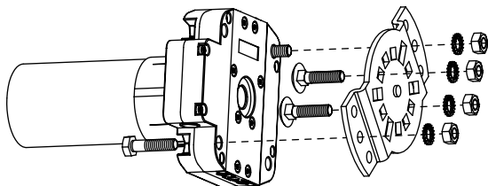
Universallager
