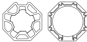
Achtkantwelle
