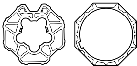
Achtkantwelle
