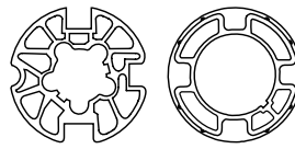
Rundwelle
